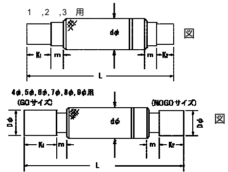
限界プラグゲージ形状及び寸法
